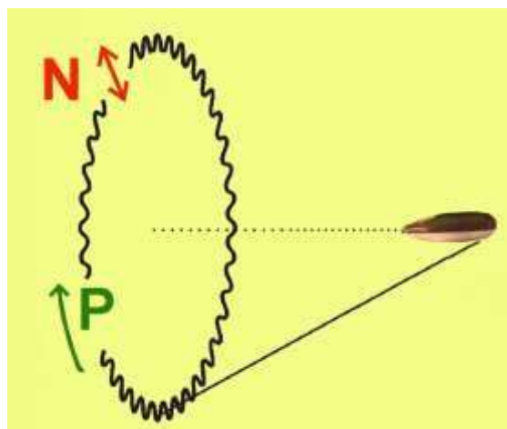
Il fenomeno di precessione e nutazione illustrato graficamente
